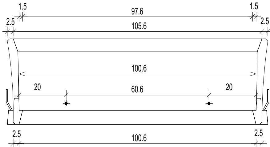
Schnitt B-B
