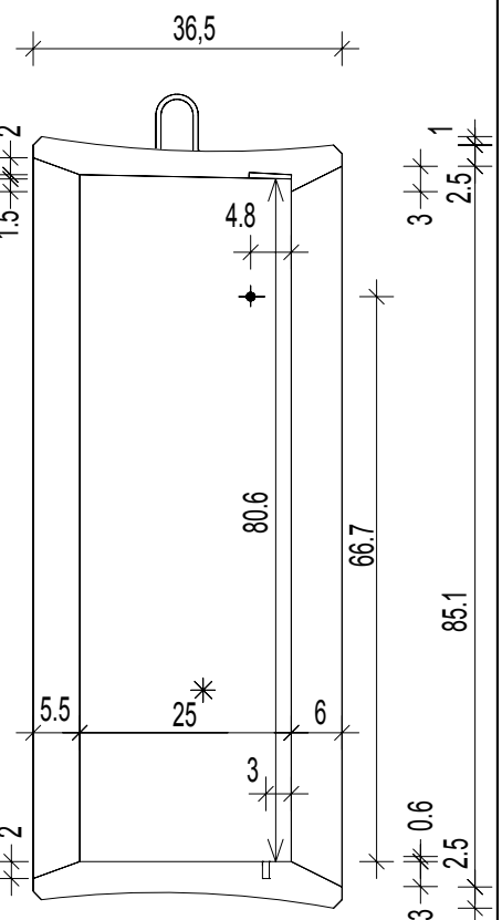
Schnitt A-A
