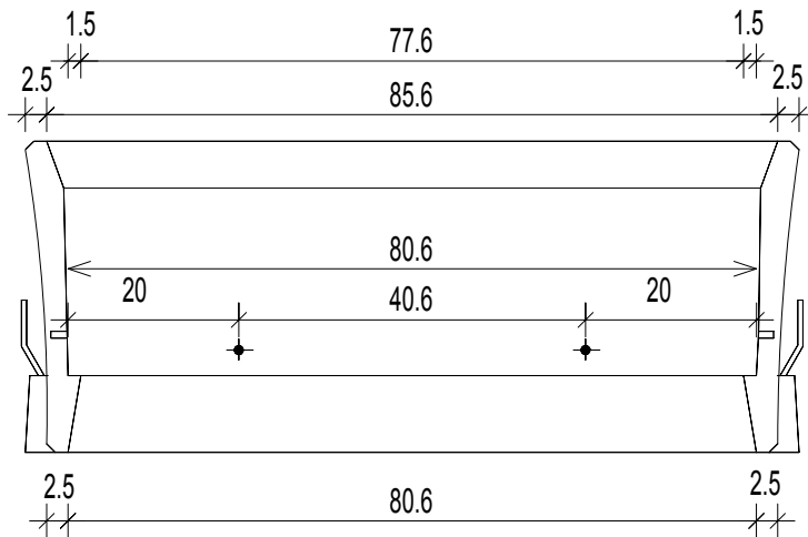
Schnitt B-B
