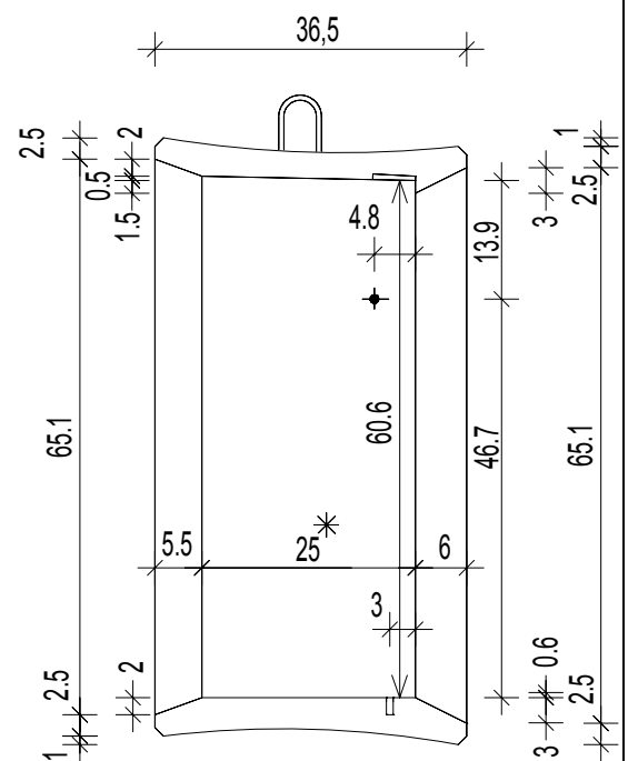
Schnitt A-A
